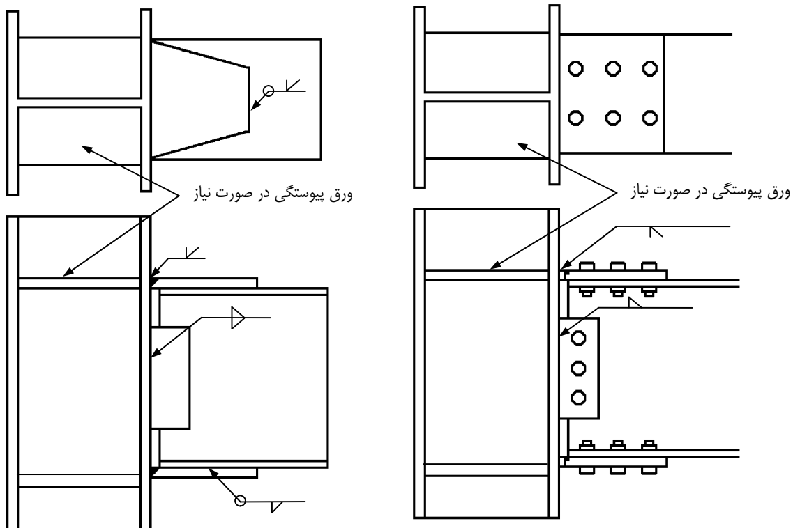
شکل (5-6-ب): اتصال ورق به بال تیر با جوش
