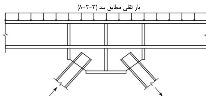
شکل (۵-۱۰): نیروی غیرمتعادل مهاربندهای کششی و فشاری
